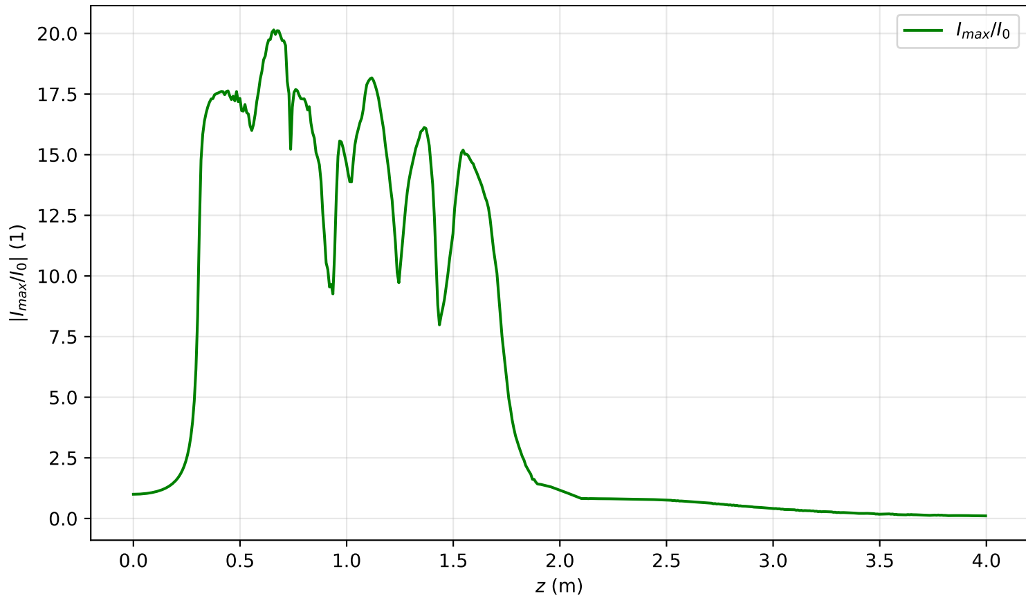
I_{max}(r=0, z)/I_0 , Pin=8.9Pcr
